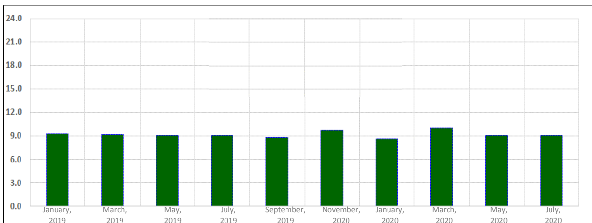
KOMPSAT-3 MTF
